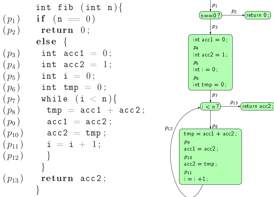
FIG. 1.2 – Un programme et son graphe de flot de contrôle condensé. Un sommet représente désormais un branchement, une jonction ou un bloc de base.
