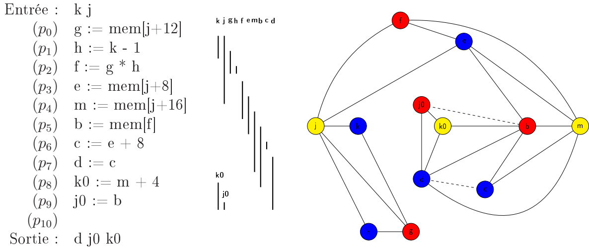
FIG. 1.13 – Le programme de référence sous forme SSA, les durées de vie de ses variables et une coloration optimale pour 3 registres ou plus. Il n'est plus nécessaire de disposer de 4 registres comme initialement car l'utilisation de la forme SSA permet aux variables k et k0 d'une part et j et j0 d'autre part d'être placées dans des registres différents.
