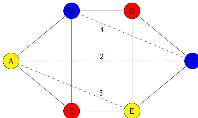
FIG. 4 – Un exemple de graphe d'interférence-affinité. Les arêtes en trait plein sont les interférences, celles en pointillés sont les affinités. La 3-coloration du graphe correspond à une allocation de registres satisfaisant les deux affinités de plus grands poids.
