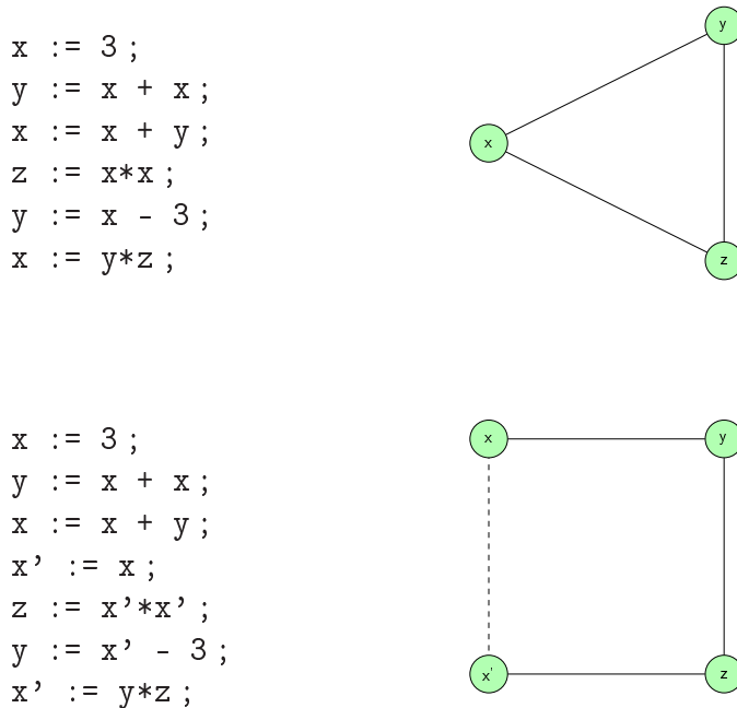
FIG. 5 – Un programme et son graphe d’interférence-affinité avant et après découpage de la durée de vie de la variable x . Avant découpage, le modèle impose de disposer de trois emplacements pour les variables du programme. Si seulement deux registres sont disponibles, l’une des trois variables est vidée en pile. Après découpage, il est tout à fait possible de stocker les trois variables dans seulement deux registres, au prix d’une instruction move supplémentaire.
