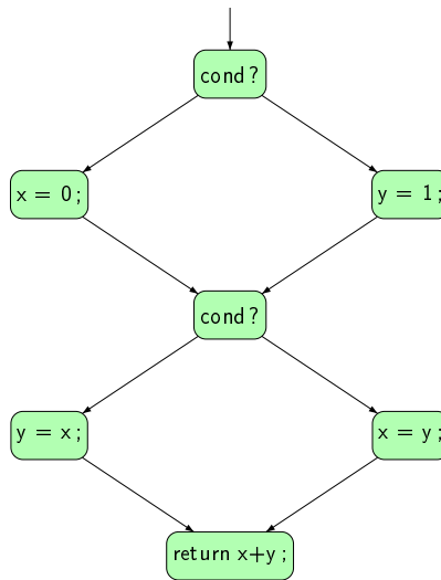
FIG. 1.4 – Un programme non strict.
