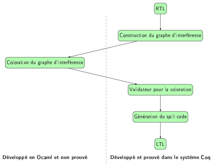
FIG. 7 – Schéma de l’allocation de registres de CompCert.
