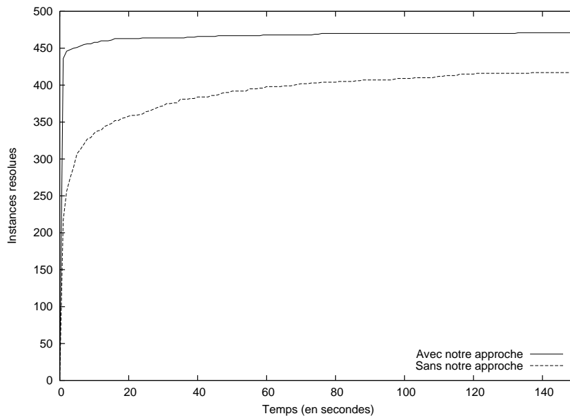
FIG. 6.6 – Nombre d'instances de l'OCC résolues en moins de 150 secondes par l'algorithme de coupes avec et sans réduction préalable.
