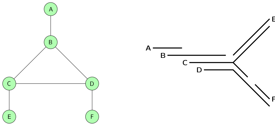
FIG. 5.5 – Un graphe triangulé et l'une de ses décompositions arborescentes. La décomposition indique que la largeur d'arbre du graphe est égale à 2, puisque la plus grande intersection ne contient que trois sous-arbres.
