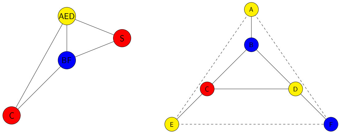
FIG. 5.16 – Le graphe fusionné de l'ensemble compatible optimal obtenu par programmation linéaire. Ce graphe est triangulé et peut, à ce titre, être facilement coloré en temps polynomial.
