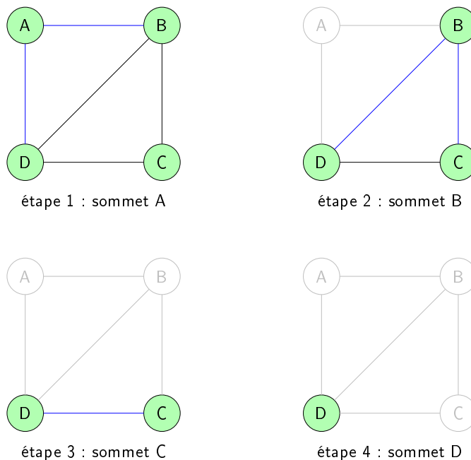
FIG. 1.15 – Un graphe triangulé et la construction d'un de ses ordres d'élimination simpliciale, l'ordre (A B C D), étape par étape.
