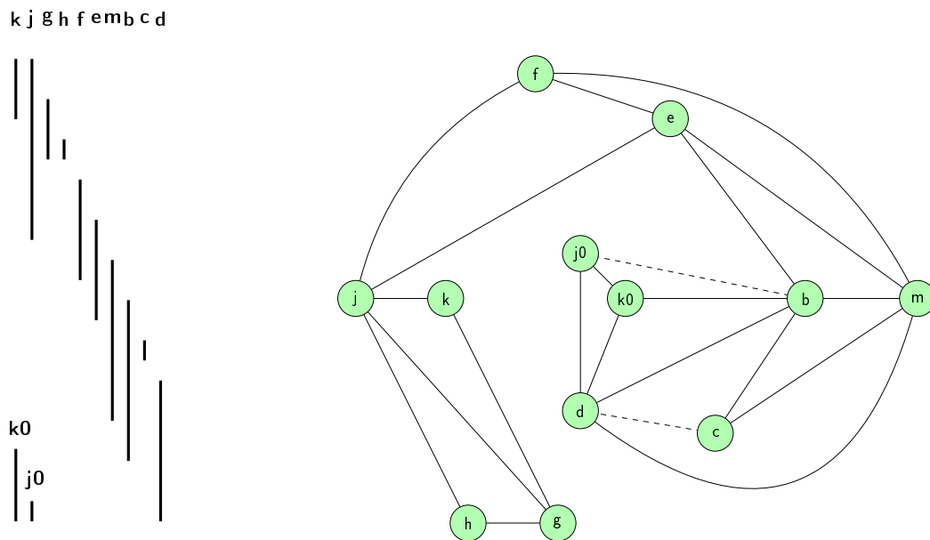
FIG. 5.16 – Le graphe fusionné de l'ensemble compatible optimal obtenu par programmation linéaire. Ce graphe est triangulé et peut, à ce titre, être facilement coloré en temps polynomial.
