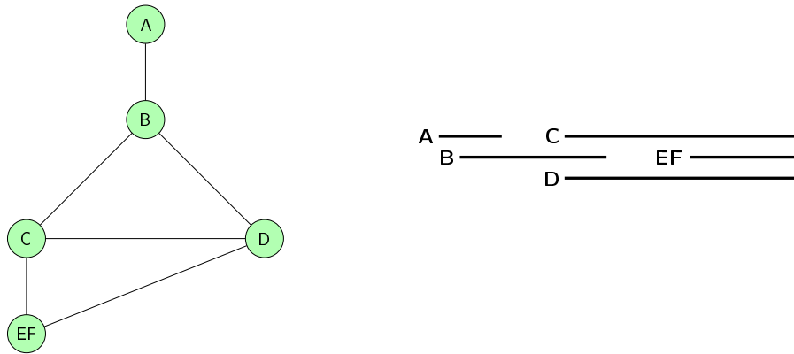
FIG. 5.10 – Le graphe obtenu après fusion de E et F dans G et la décomposition arborescente construite comme décrit durant la preuve du lemme 21.
