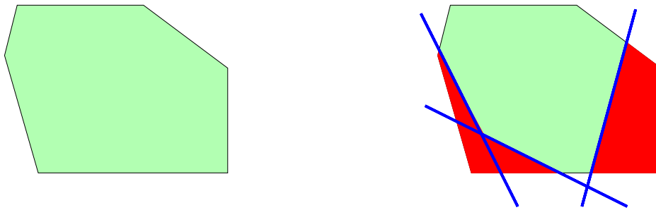
FIG. 1.10 – Schématisation de l'effet des coupes (en bleu) sur la région admissible de la relaxation continue (en vert). La zone rouge correspond à la partie de la région admissible pour la relaxation continue ne respectant pas les coupes.
