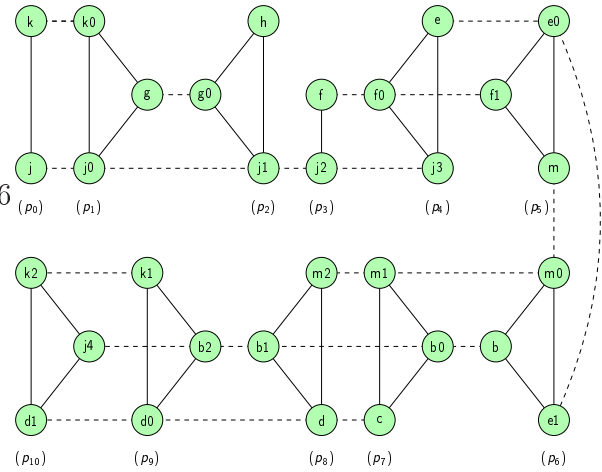
FIG. 1.19 – Le programme de référence, son graphe d'interférence-affinité, sa forme élémentaire telle que définie par Appel et George et son graphe éclaté.
