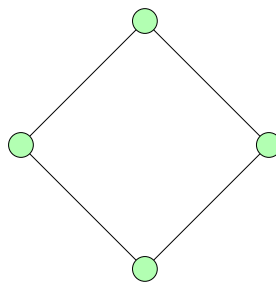
FIG. 1.8 – Un exemple de graphe simple pour lequel l’heuristique de Chaitin génère un stockage en pile inutile, pour K = 2 . Aucun sommet n’est trivialement colorable puisque chaque sommet est de degré 2. En revanche l’intégration du vidage optimiste remédie au problème.
