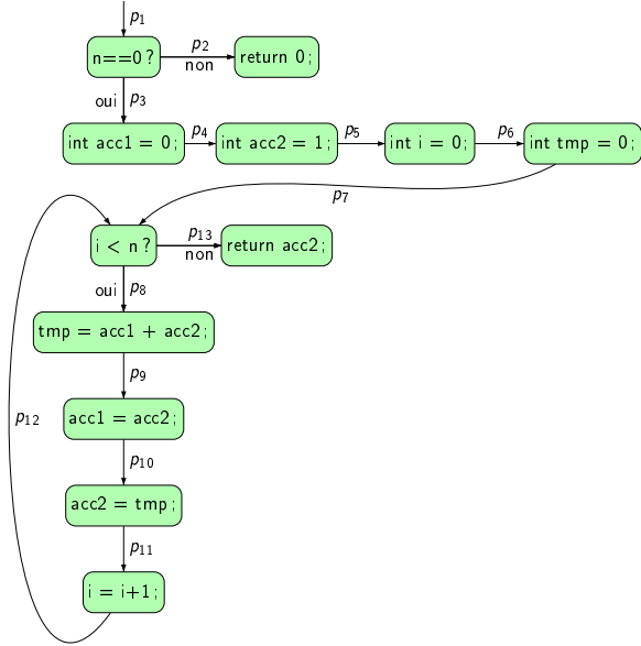
FIG. 1.1 – Un programme et son graphe de flot de contrôle.
