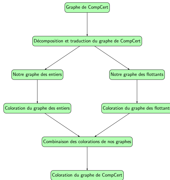
FIG. 3.6 – Description de l’intégration de notre allocateur de registres au sein de CompCert.
