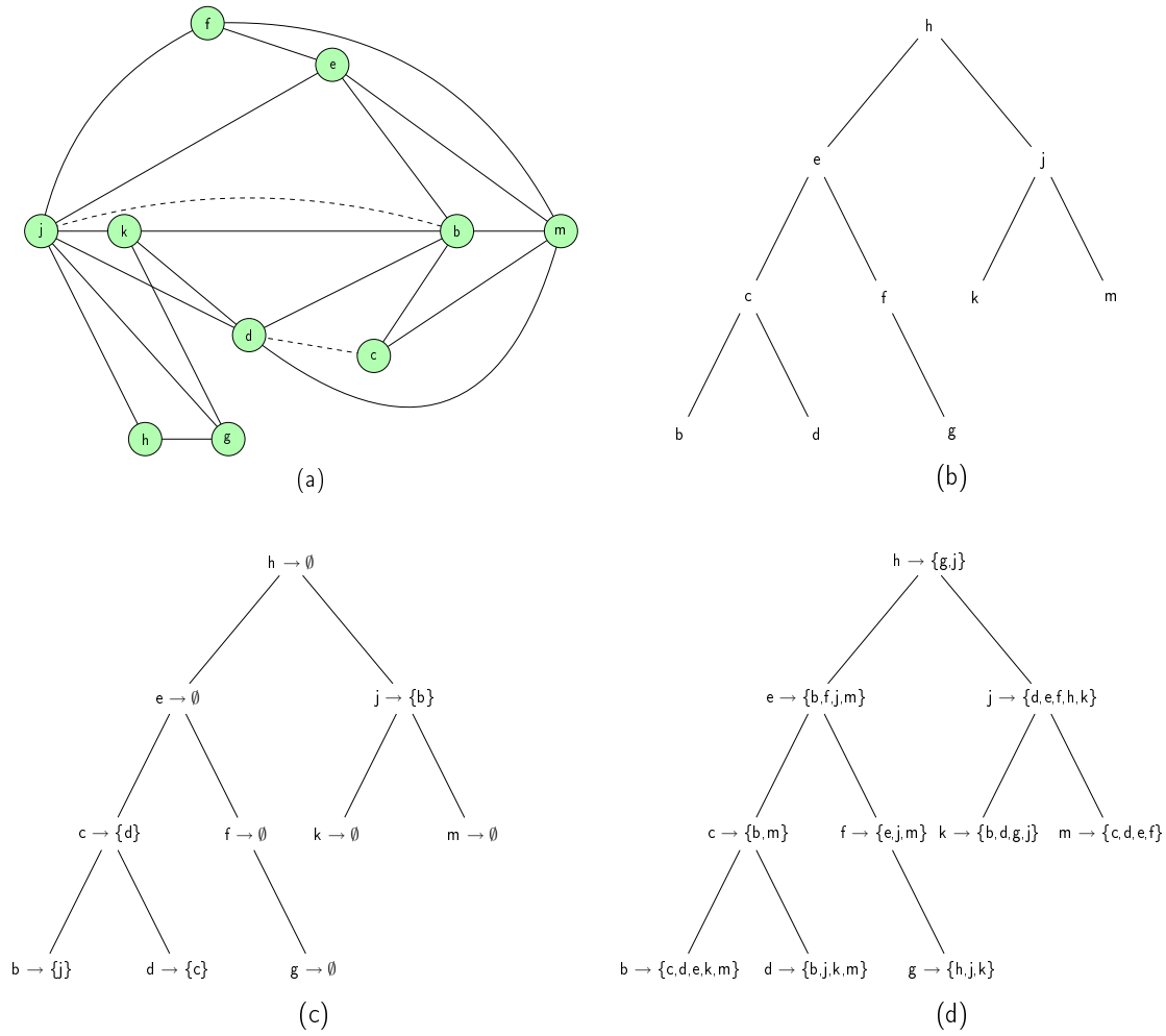
FIG. 2.7 – Un graphe (a), l'arbre AVL des sommets du graphe (b), l'arbre AVL des affinités du graphe (c) et l'arbre AVL des interférences du graphe (d). Les ensembles notés entre accolades correspondent à des ensembles qui sont également représentés par des arbres AVL, mais que nous n'avons pu exhiber sous cette forme ici pour des raisons de lisibilité.
