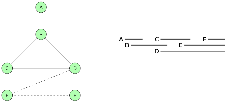
FIG. 5.9 – Une triangulation G' de G (défini figure 5.8) et une décomposition arborescente de G' de largeur d’arbre 2.
