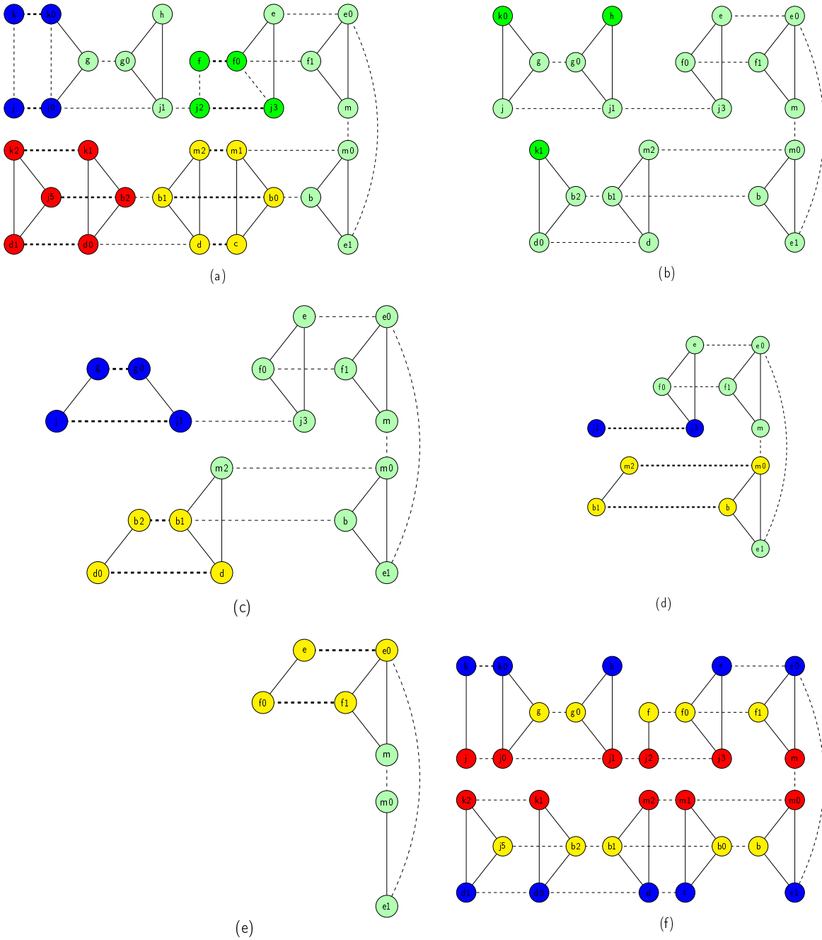
FIG. 6.3 – Application de la recomposition à l'exemple. Les couplages asservissant sont en gras à chaque itération.
