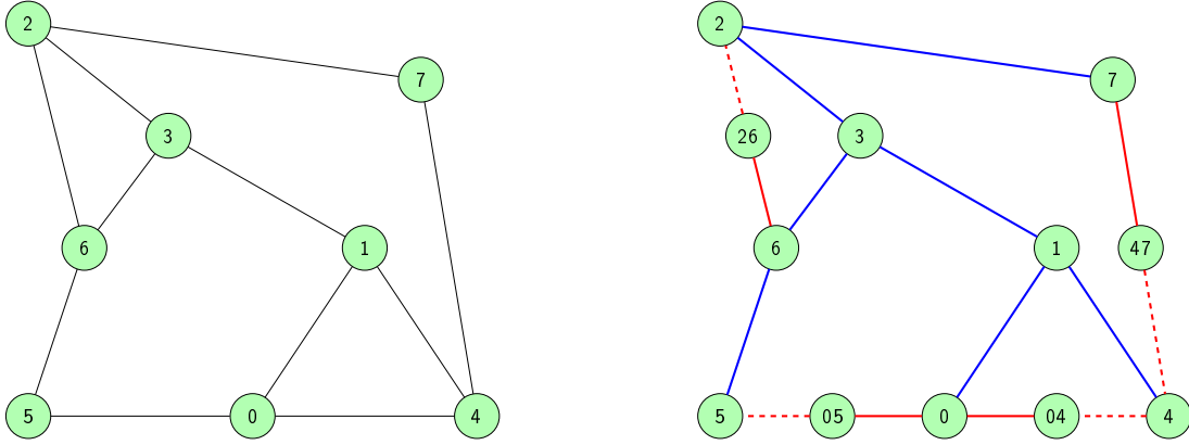
FIG. 5.1 – Exemple de construction de G' (à droite) à partir de G (à gauche). Les arêtes de l'arbre couvrant T sont en bleu tandis que les arêtes ajoutées lors de la réduction sont en rouge.
