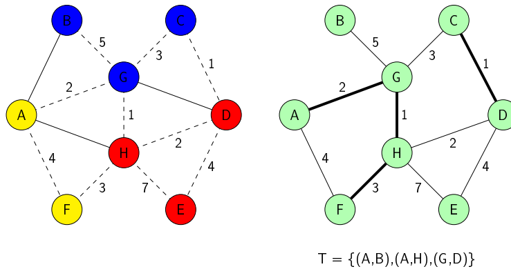
FIG. 5.6 – Un graphe d’interférence-affinité G et MC(G) . Le graphe est pourvu d’une 3-coloration optimale. Les arêtes en gras forment une multicoupe optimale et correspondent exactement aux affinités non satisfaites dans G .
