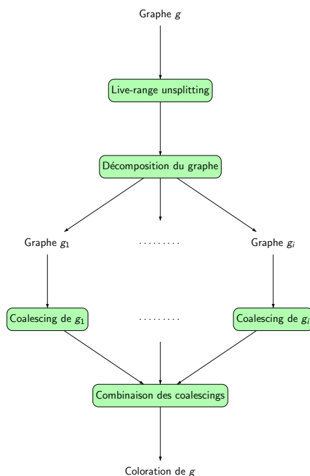
FIG. 6.4 – Le processus complet de fusion.
