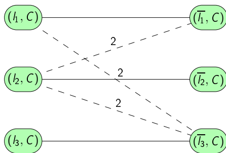
FIG. 5.2 – Le premier gadget. Si on ne considère que 2 couleurs, ce gadget rapporte une valeur d'affinité nulle si tous les sommets de gauche ont la même couleur et une valeur d'affinité de 4 sinon.
