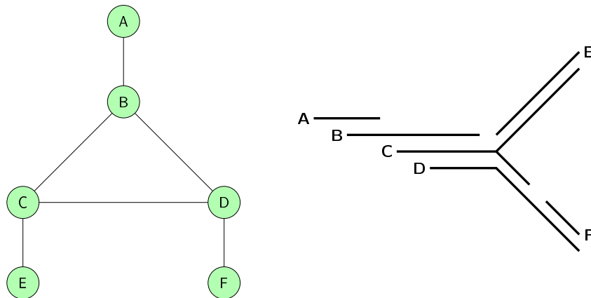
FIG. 1.16 – Un graphe triangulé et une représentation en tant que graphe d'intersection des sous-arbres d'un arbre.
