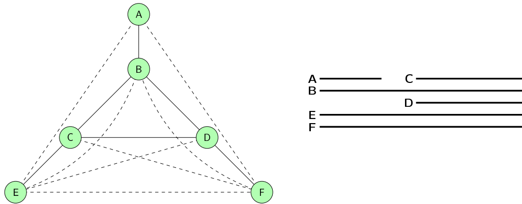
FIG. 5.13 – Une triangulation G'' et une décomposition arborescente du graphe G'' .
