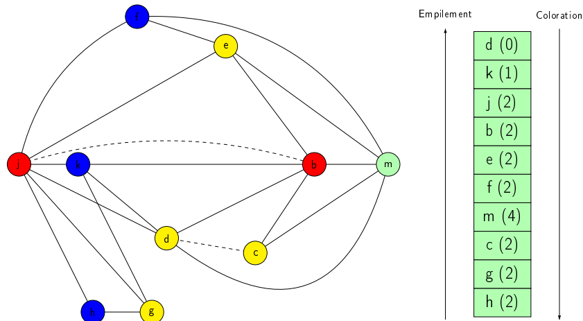
FIG. 1.7 – Illustration de l’heuristique de vidage de Chaitin pour K = 3 . Les degrés indiqués à côté de la pile sont les degrés d’interférence des sommets au moment de leur empilement. Un degré d’interférence supérieur ou égal à K signifie que la variable est vidée en pile.
