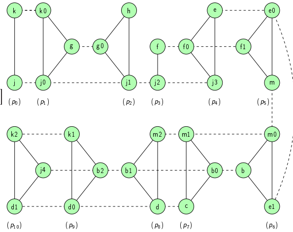
FIG. 6.1 – Le programme de référence, son graphe d’interférence-affinité et son graphe éclaté. Le graphe éclaté donne une bonne représentation du flot de données du programme.
