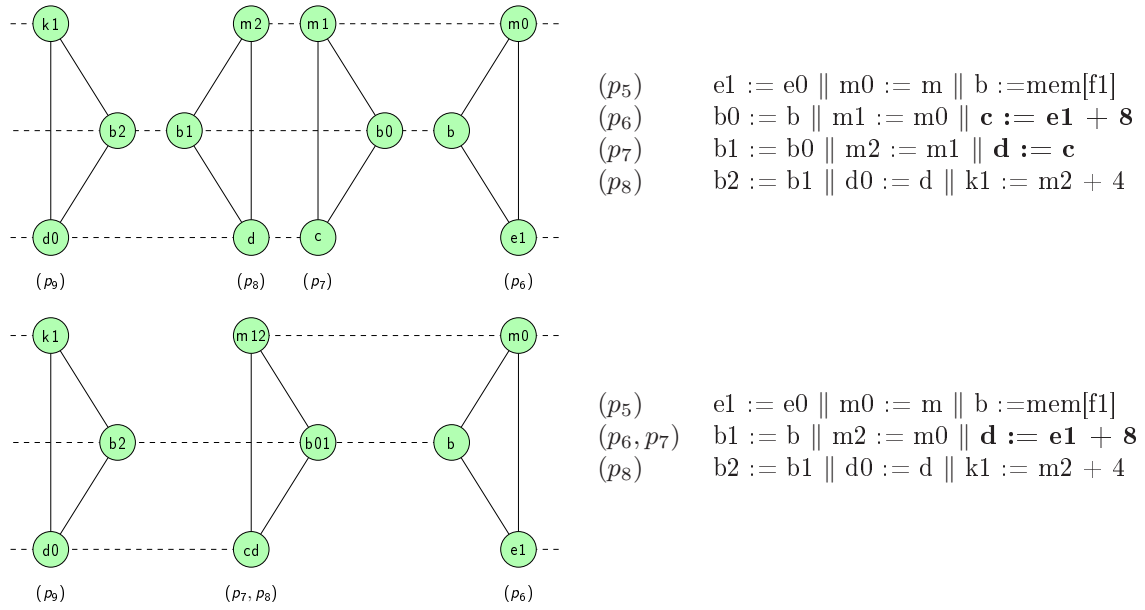
FIG. 6.2 – En haut, deux cliques parallèles et le morceau de programme correspondant. En bas, le même sous-graphe et son code correspondant après une étape de recombinaison.
