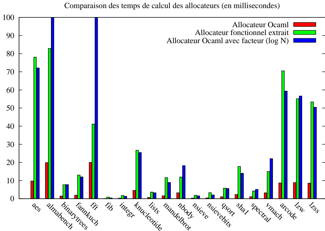
FIG. 3.8 – Comparaison des temps pris par chacun des allocateurs de registres. Afin d’améliorer la lecture, les résultats pour les instances almabench et fft sont tronqués à 100 millisecondes dans la troisième colonne alors que ceux-ci s’élèvent respectivement à 131 et 120 millisecondes.
