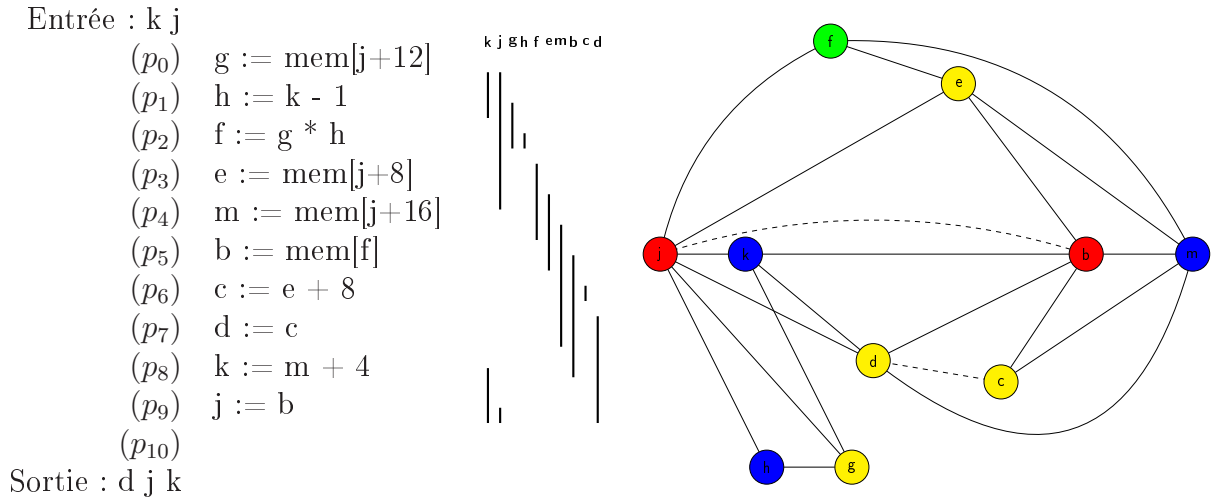
FIG. 1.5 – Un programme, les durées de vie de ses variables, et son graphe d'interférence-affinité. Les variables k et j sont supposées vivantes en entrée et les variables d, k et j sont supposées vivantes en sortie. La coloration du graphe d'interférence-affinité proposée est optimale pour quatre registres ou plus, puisque chaque sommet est coloré et que les deux affinités sont satisfaites.
