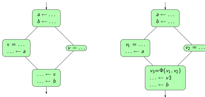
FIG. 1.14 – Un programme et sa forme SSA. Une \Phi -fonction est ajoutée à la jonction afin d'unifier les différentes copies de la variable v .
