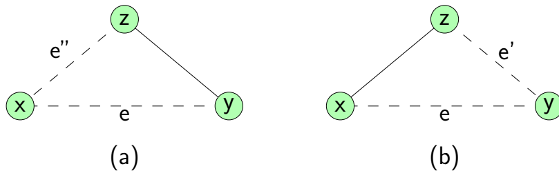
FIG. 2.4 – Deux configurations menant à la disparition d'une affinité au profit d'une interférence après fusion de x et y . Avant fusion x et z sont liés par une affinité dans le cas (a) et par une interférence après fusion. Dans le cas (b), ce sont y et z qui sont liés par une affinité qui est éclipée par l'interférence entre x et z après la fusion.
