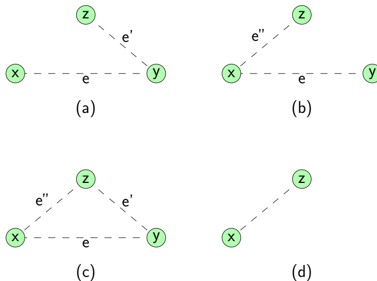
FIG. 2.5 – Trois configurations (a), (b) et (c) menant à une configuration identique (d) après fusion de x et y .
